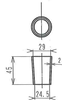
テーパ管詳細図
